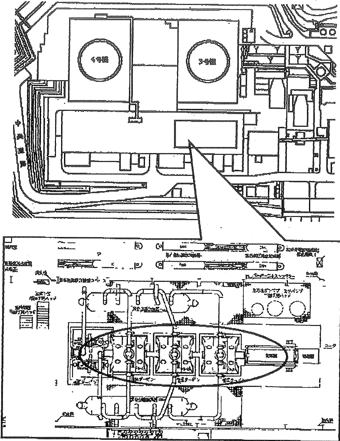
3号機 タービン建屋 EL21.8m タービン
