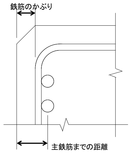
図3-4 鉄筋のかぶり
