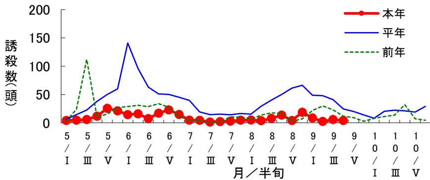
黄色水盤によるアブラムシ類誘殺数の推移(飛騨市古川町)
