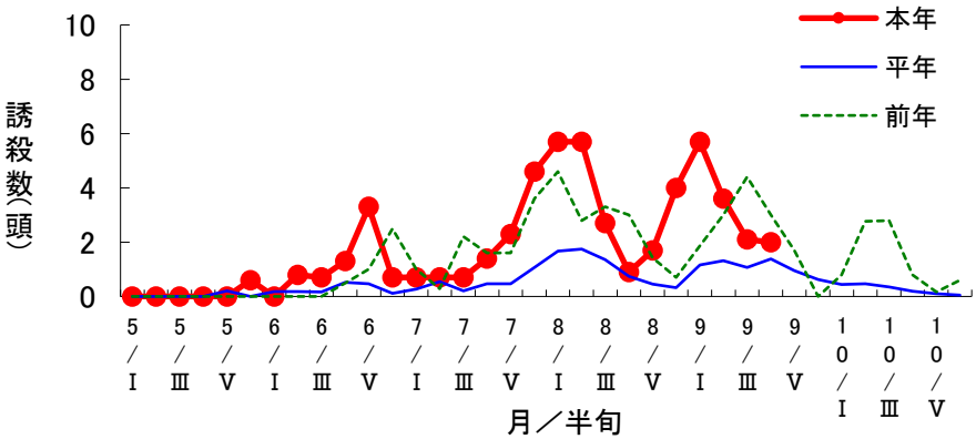
フェロモントラップによるタバコガ誘殺数の推移(下呂市御厩野)
