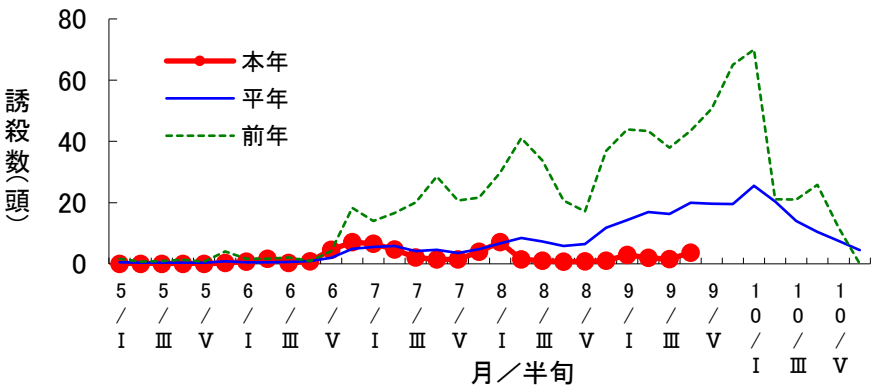
フェロモントラップによるオオタバコガ誘殺数の推移(下呂市御厩野)
