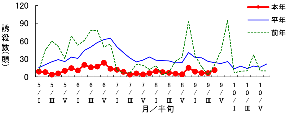
黄色水盤によるアブラムシ類誘殺数の推移(下呂市御厩野)
