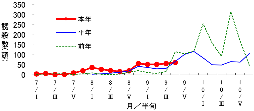
フェロモントラップによるハスモンヨトウ誘殺数の推移(飛騨市古川町)
