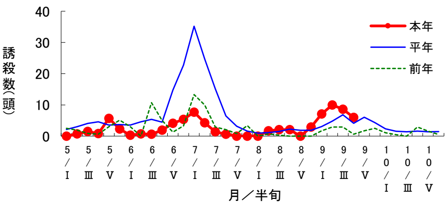
誘引物質によるタネバエ誘殺数の推移(飛騨市古川町)
