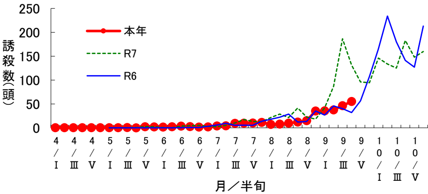
フェロモントラップによるトマトキバガ誘殺数の推移(飛騨市古川町)
