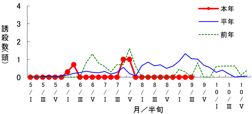
フェロモントラップによるタバコガ誘殺数の推移(高山市丹生川町)
