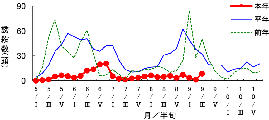
黄色水盤によるアブラムシ類誘殺数の推移(高山市下林町)
