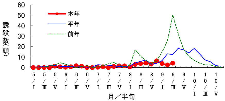
フェロモントラップによるオオタバコガ誘殺数の推移(高山市丹生川町)
