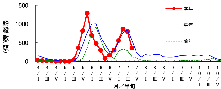
フェロモントラップによるチャノホソガ誘殺数の推移(池田町般若畑)
