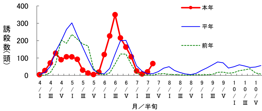
フェロモントラップによるチャノコカクモンハマキ誘殺数の推移(池田町般若畑)
