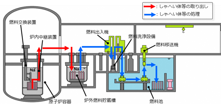
しゃへい体等取出し作業の流れ
