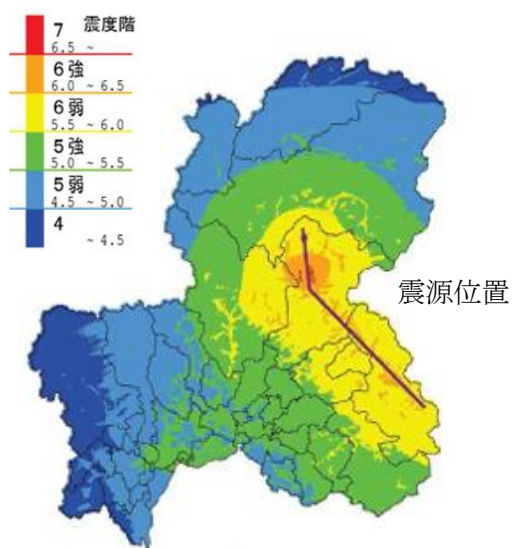
阿寺断層系地震の震度予測
