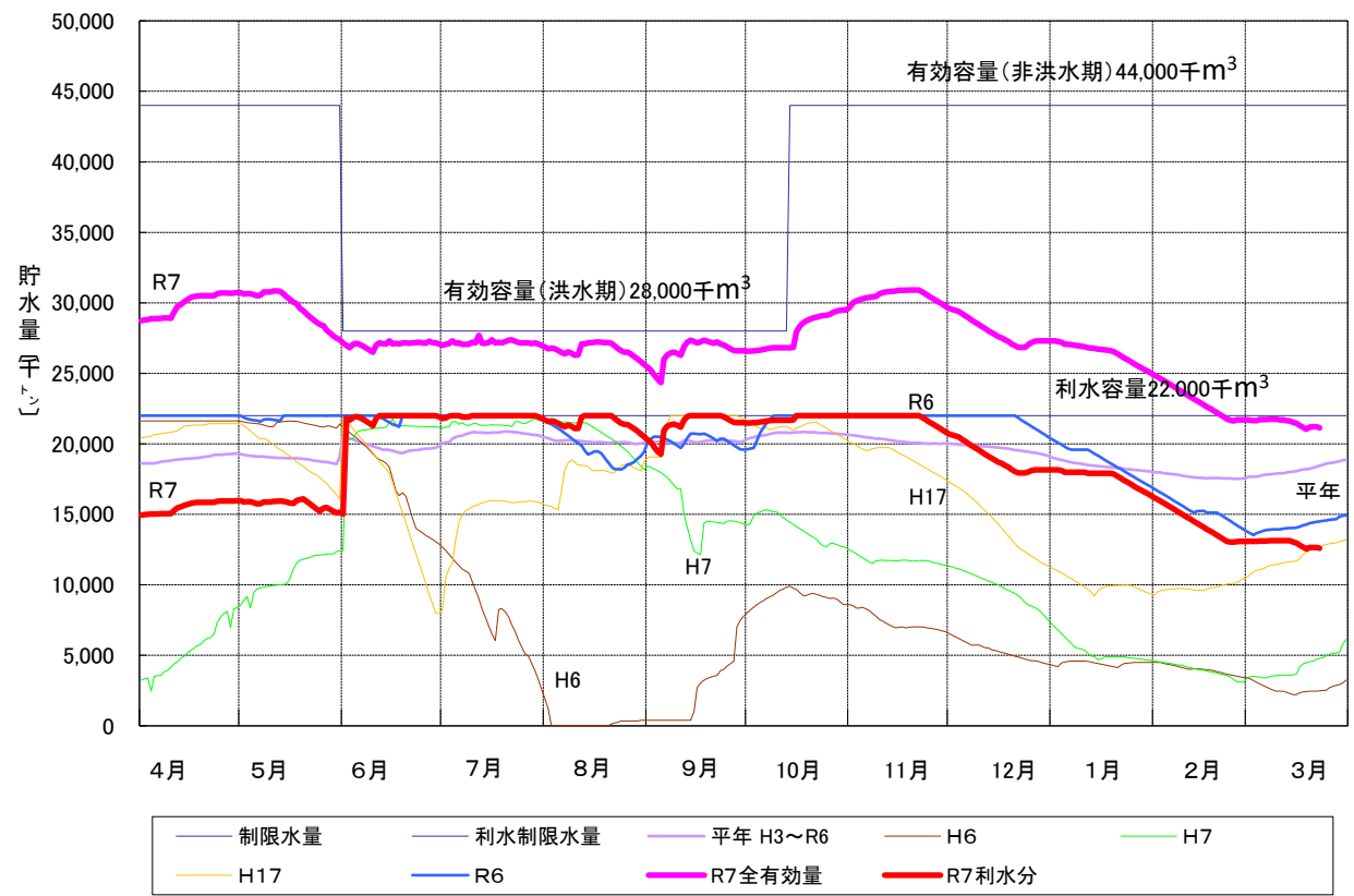
阿木川ダム貯水運用曲線
