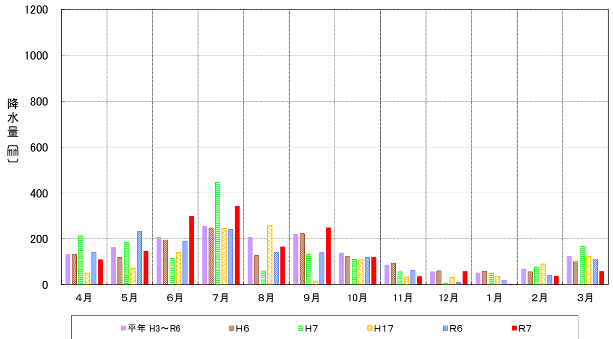
阿木川ダム降水量
