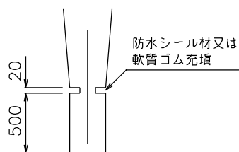
図 12.2.12 ヒンジ構造
