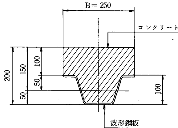
図 12.2.19 合成版の構造
