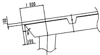
図 12.2.11 底形状
