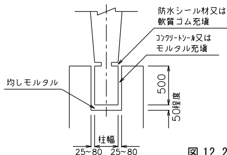
図 12.2.13 柱受構造
