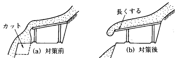
図 12.2.3 沈降力の対策例
