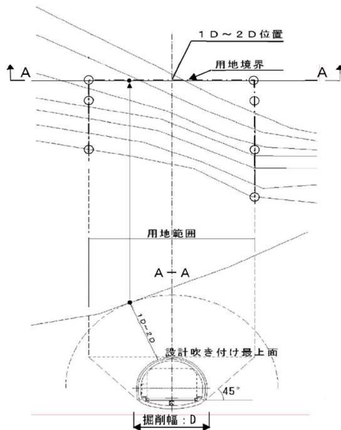
図 1.23 坑口部の用地取得範囲
