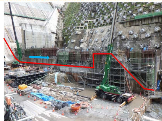
減勢工(下流側から望む)
