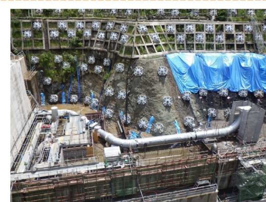
発電所水圧管
