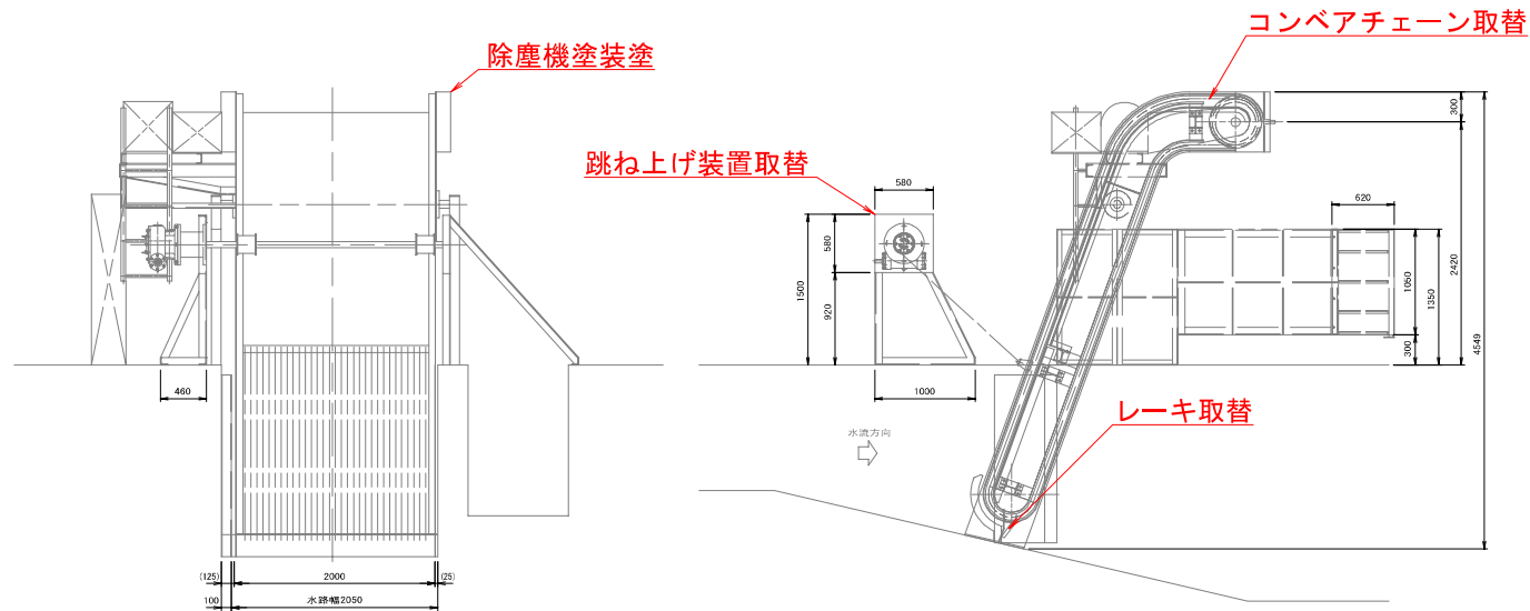
正面図
