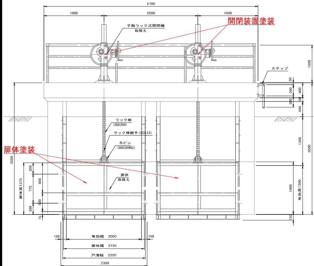
正面図
