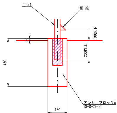
断面図
