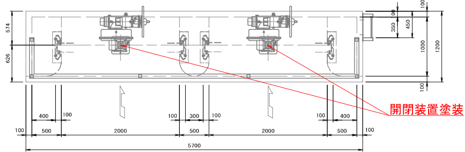
平面図
