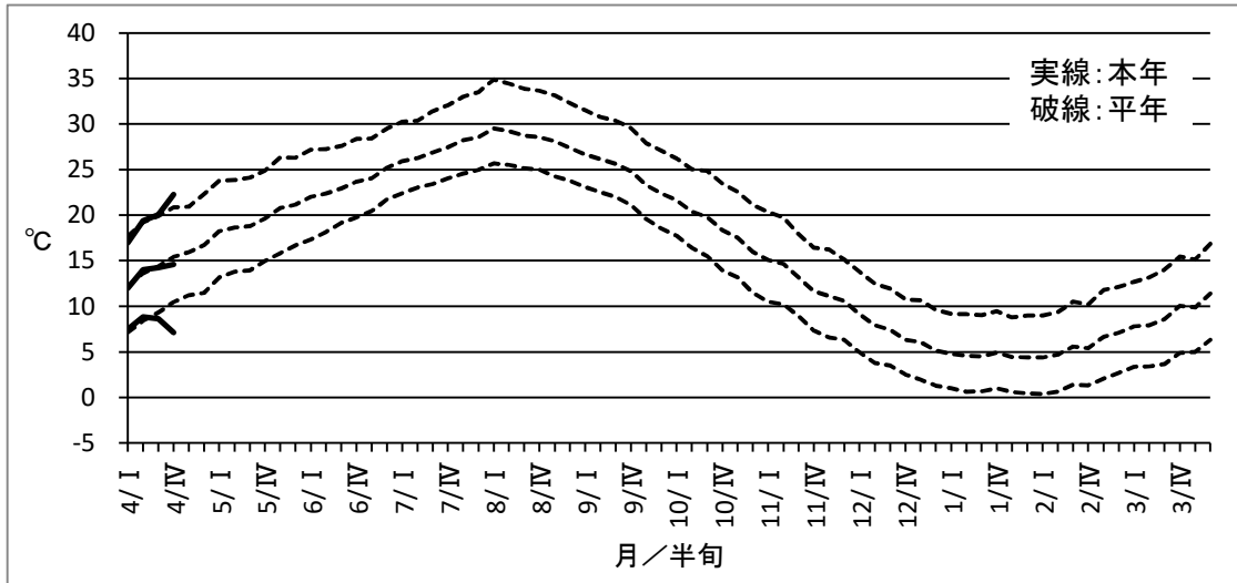
令和7年度気象グラフ(観測地点:岐阜市) 気温(半旬平均)
