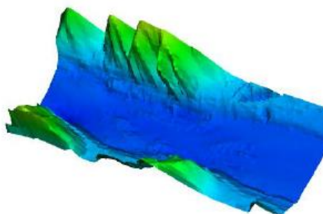
図- 2.8 航空レーザ測深（ALB）の計測イメージ及び河道の三次元計測データ
