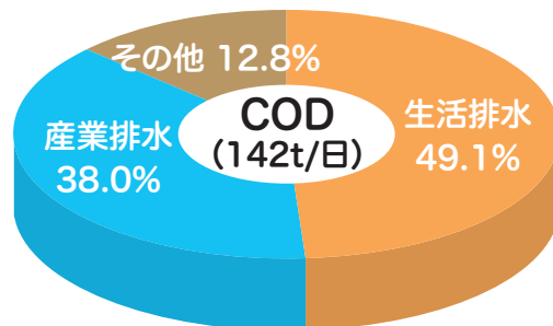
伊勢湾のCOD負荷量構成比
