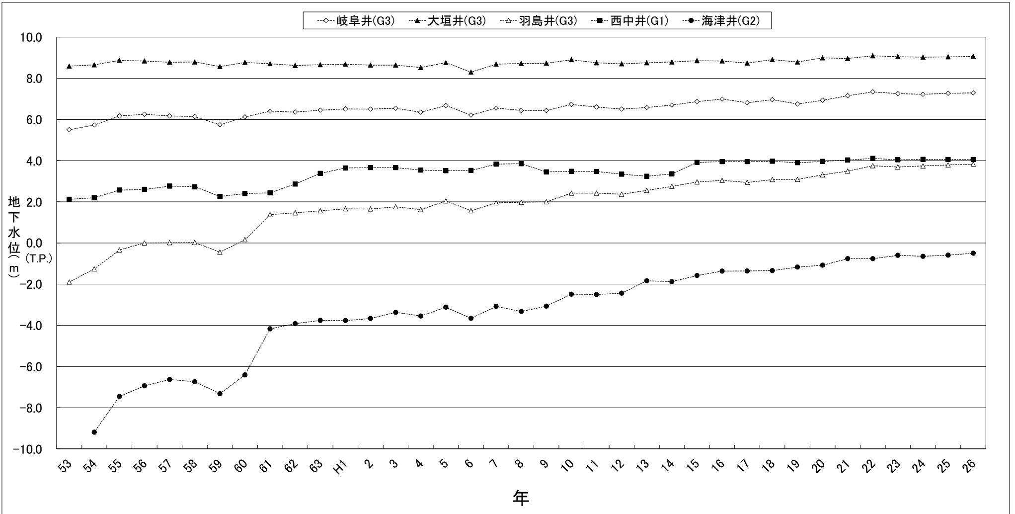
図2 主な観測井の年平均地下水位の状況
