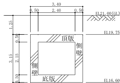
1号機LOT連絡ダクト
