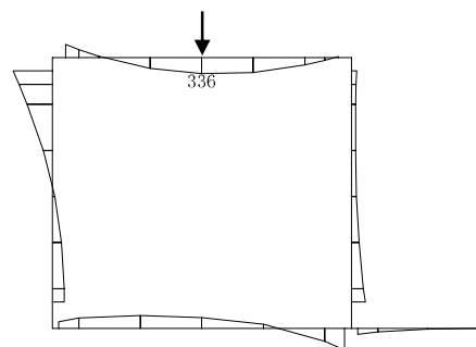
曲げモーメント(単位: \text{kN}\cdot\text{m}/\text{m} )
