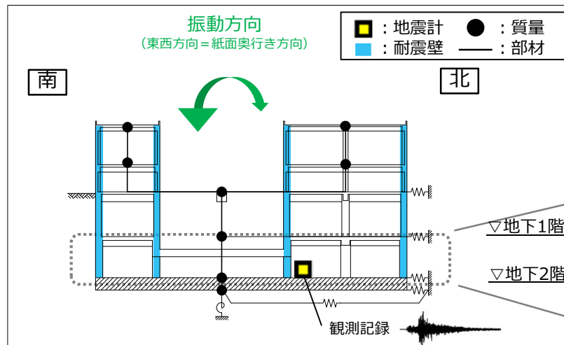
解析のイメージ（2号海水熱交換器建屋東西方向の例）
