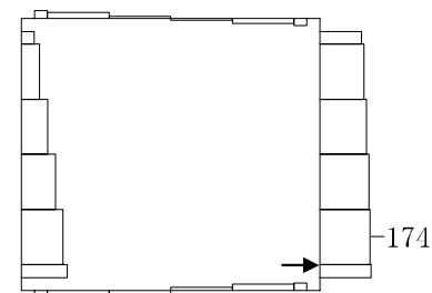
軸力※(単位:kN/m)
