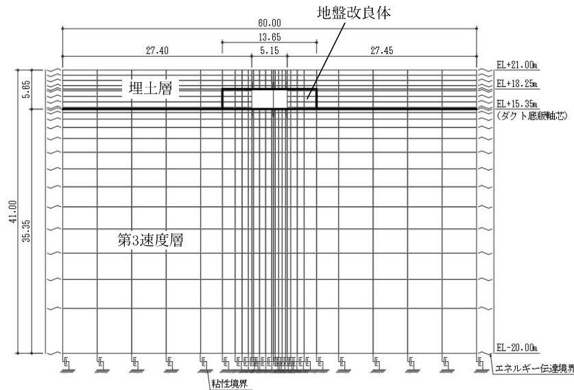
1号機SGTS連絡ダクト
