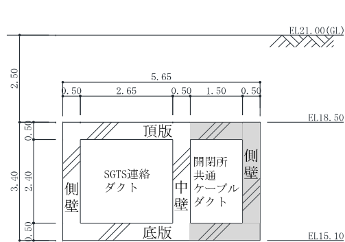
1号機SGTS連絡ダクト
