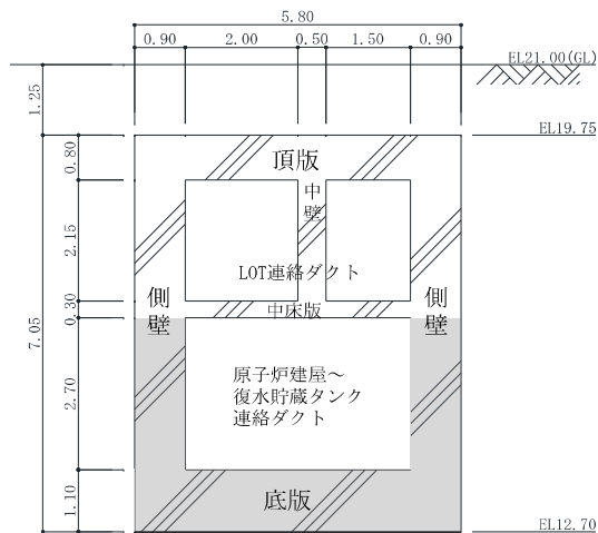
2号機LOT連絡ダクト(NS断面)
