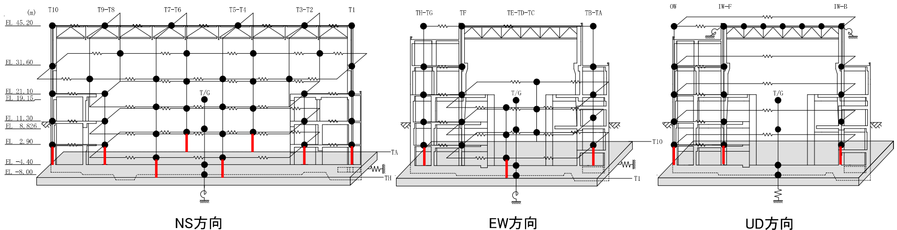
2号機タービン建屋 地震応答解析モデル※
