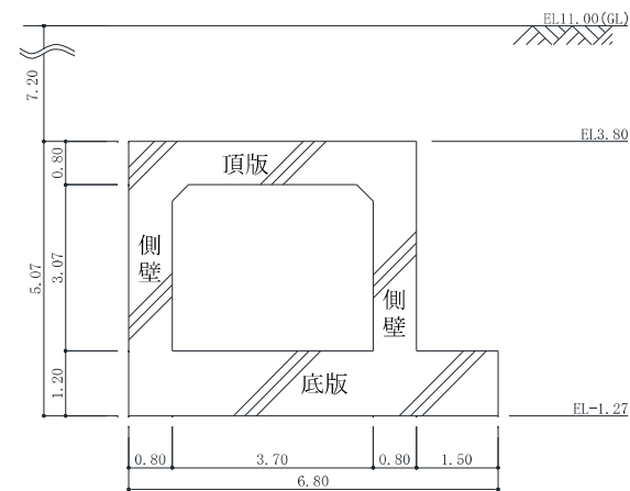
1号機RCW連絡ダクト
