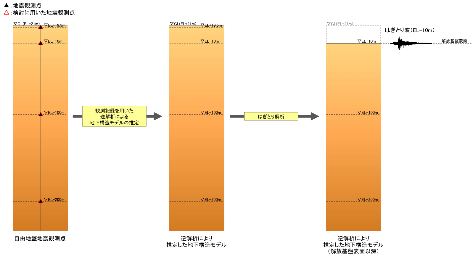
はぎとり解析の概要
