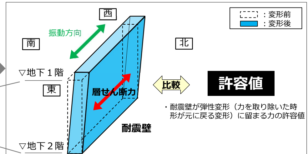
海水熱交換器建屋の耐震健全性の確認のイメージ（地下2階の例）
