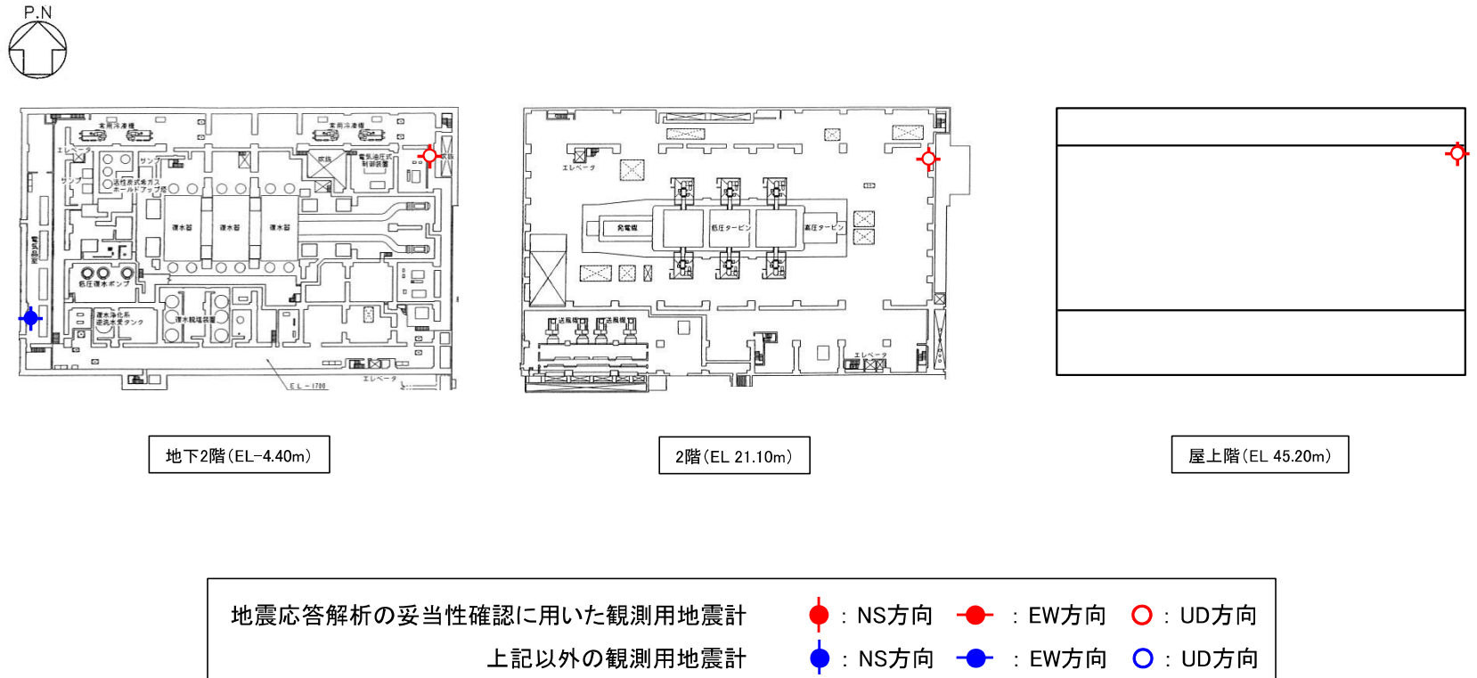
2号機タービン建屋に設置している観測用地震計の位置
