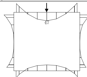
曲げモーメント(単位: \text{kN}\cdot\text{m}/\text{m} )
