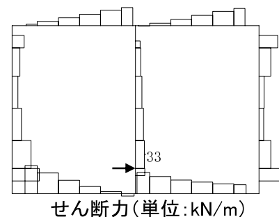
2号機LOT連絡ダクト(EW断面)
