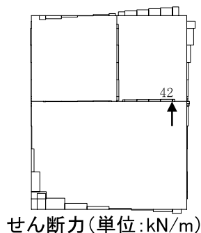
2号機LOT連絡ダクト(NS断面)
