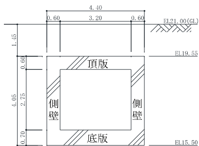
2号機SGTS連絡ダクト
