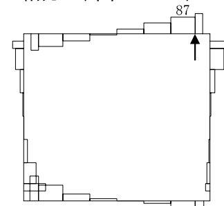
せん断力(単位: \text{kN}/\text{m} )
