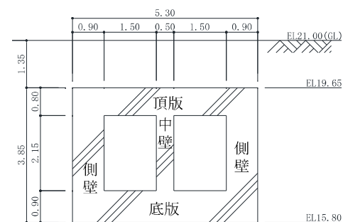
2号機LOT連絡ダクト(EW断面)
