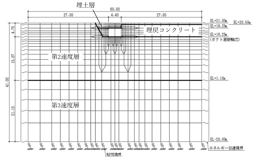
2号機LOT連絡ダクト(EW断面)
