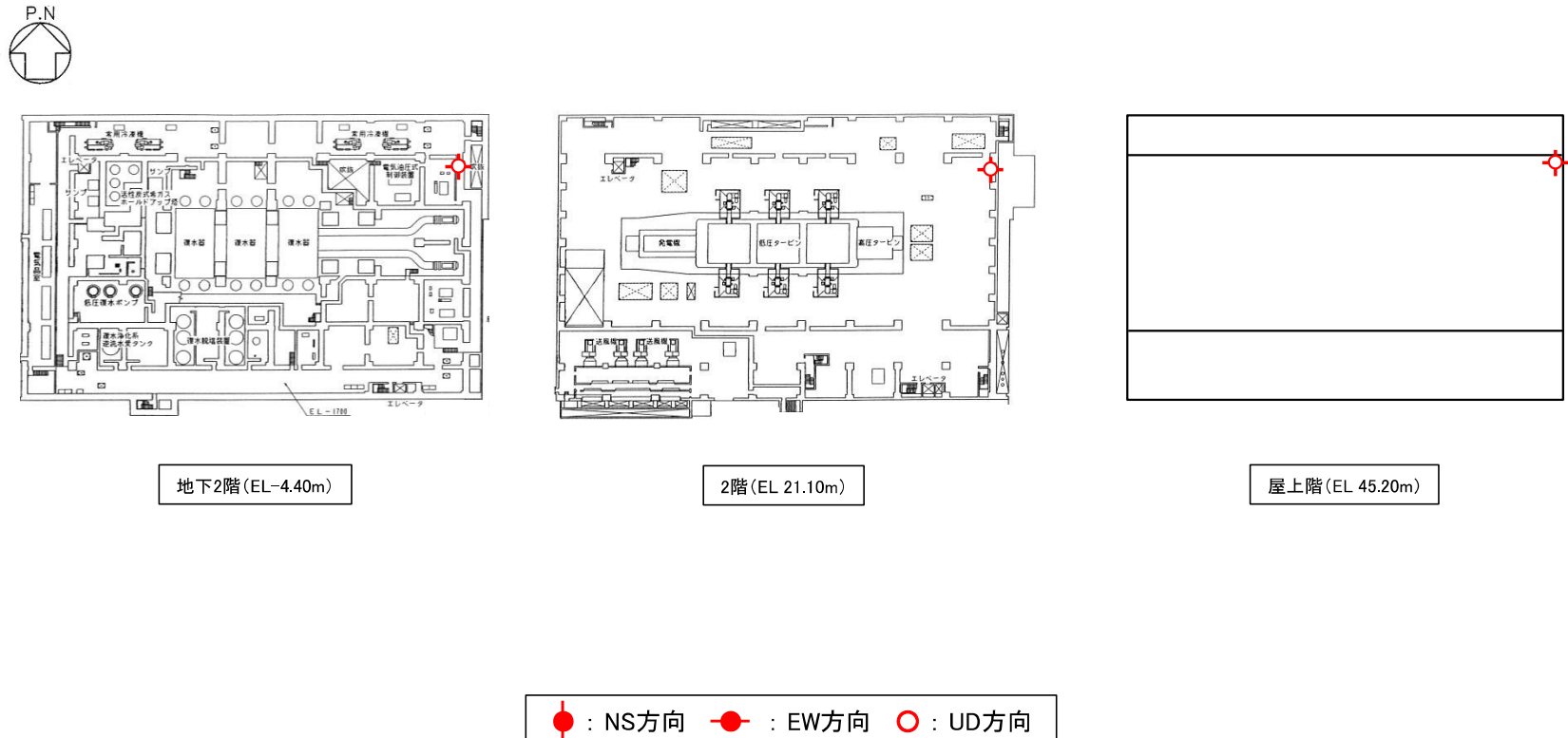
2号機タービン建屋の地震応答解析の妥当性確認に用いる観測用地震計の設置位置
