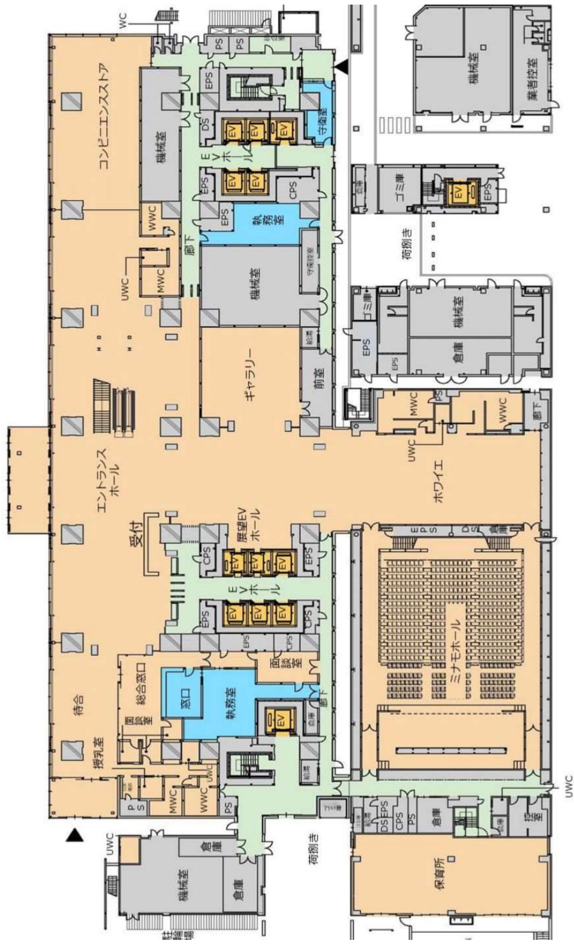
ミニモホール図面（県庁舎 1階平面図）
