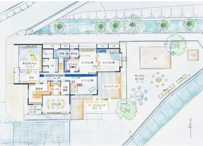
1階平面図
