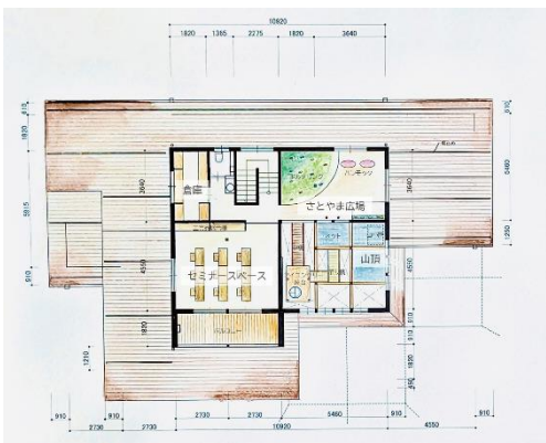
2階平面図
