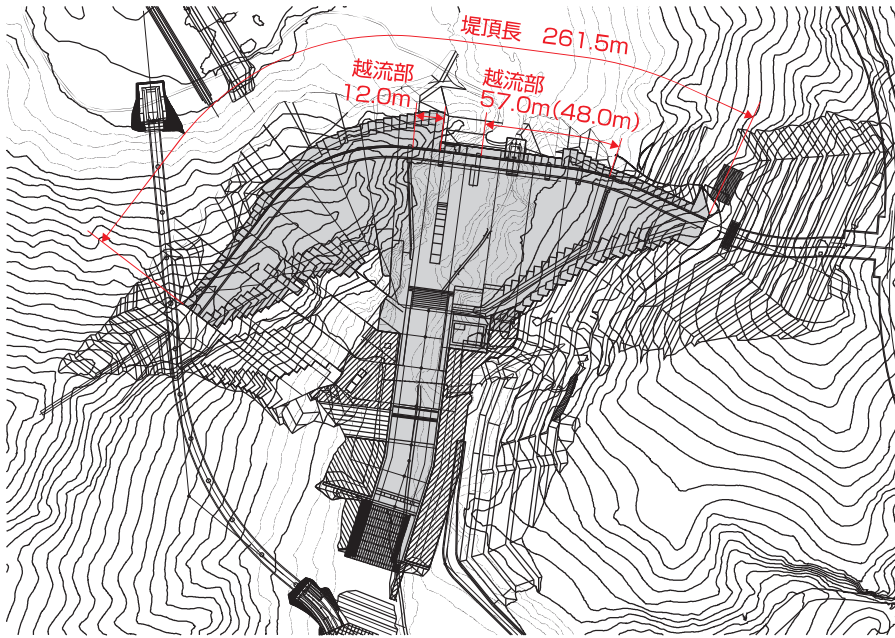
■ダム平面図
