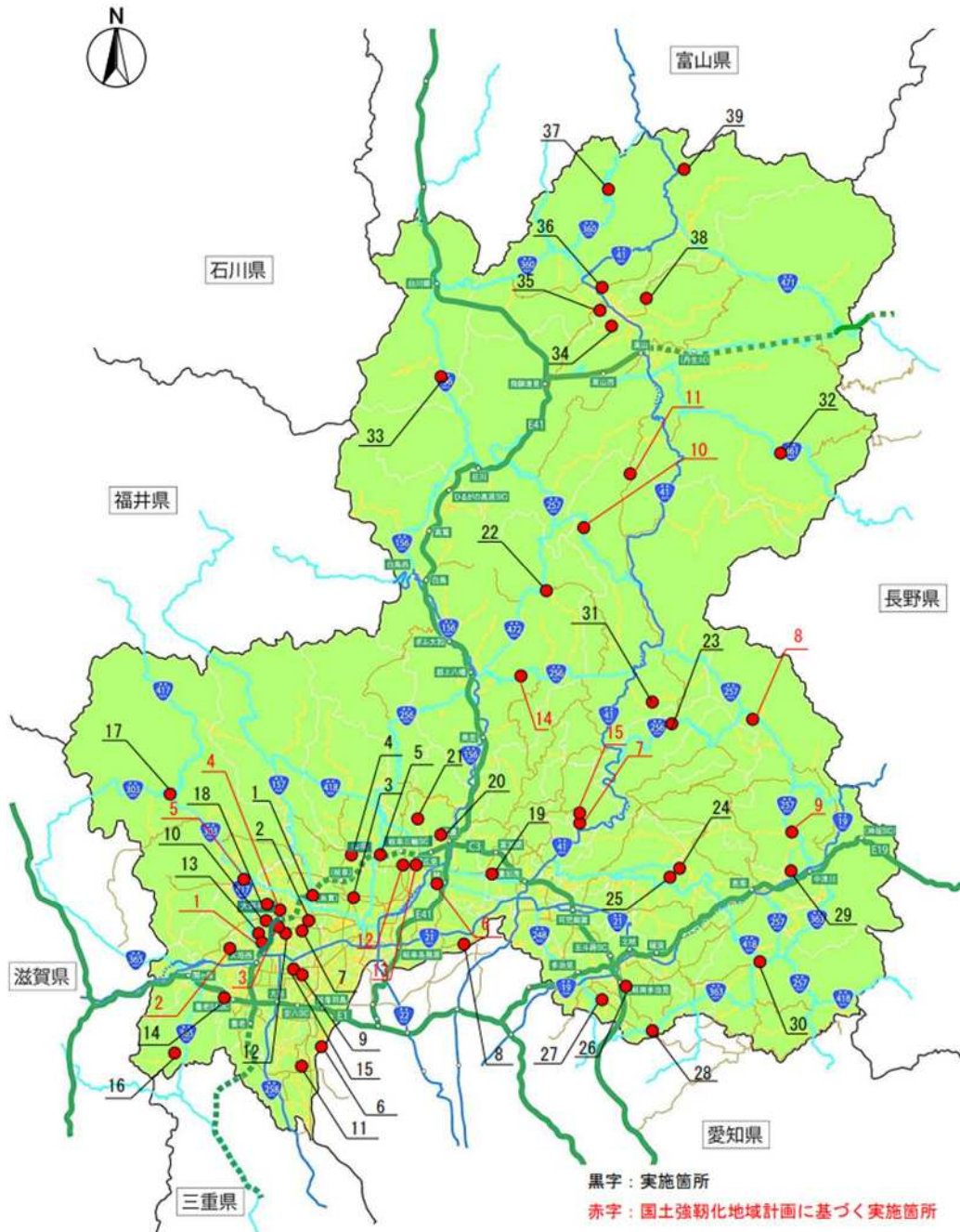
岐阜県道路整備アクションプログラム 実施箇所位置図(岐阜県事業 道路改築事業)
