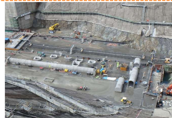
監査廊の設置状況
