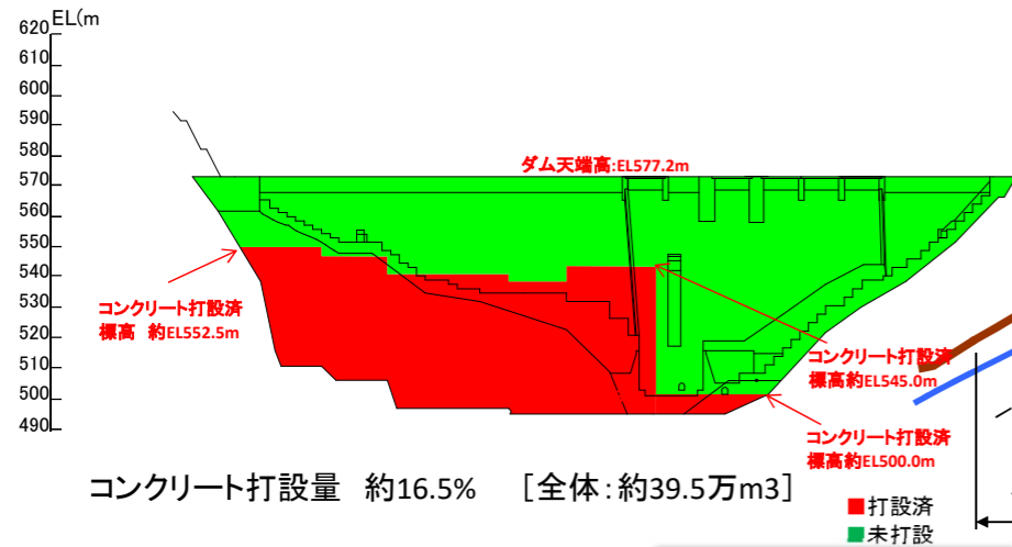
コンクリート打設進捗状況(R3.11末時点)
