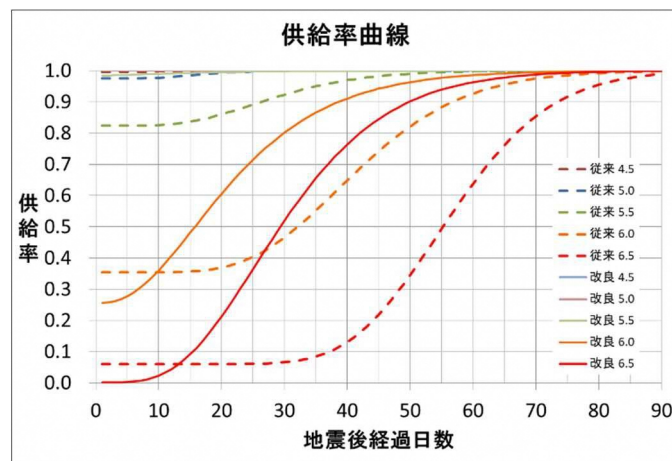
図 2-3 都市ガスの地震後経過日数と供給率
