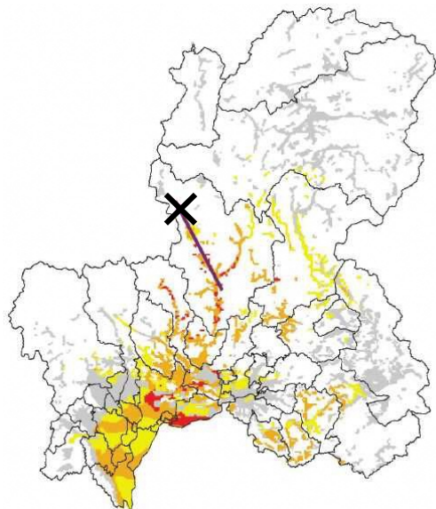
図-15 長良川上流断層帯地震（北 南）PL 値分布
