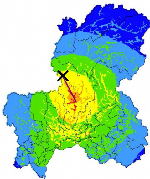
図-4 長良川上流断層帯地震（北 南）震度階分布
