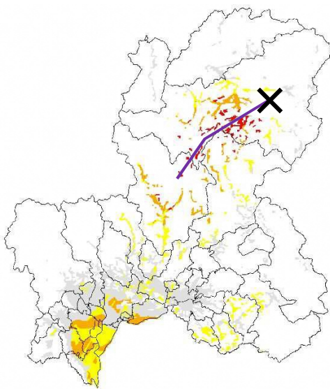
图-20 跡津川断層地震(北東 南)PL 值分布
