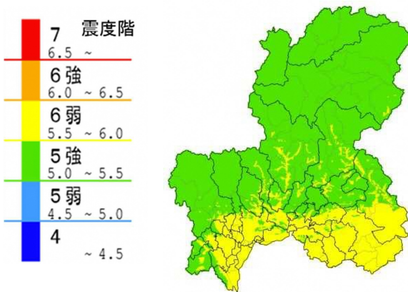
図-1 南海トラフの巨大地震震度階分布
