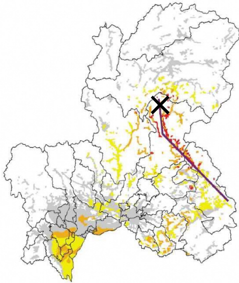
图-18 阿寺断層系地震（北 南東）PL 值分布
