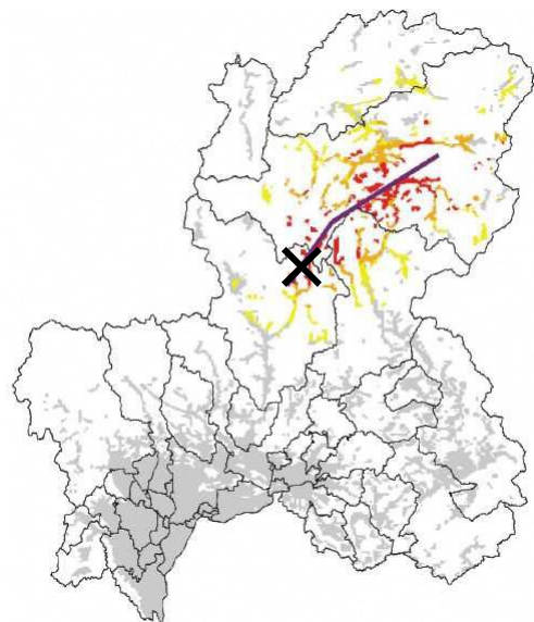
图-22 高山・大原断層帯地震（南 北東）PL 值分布
