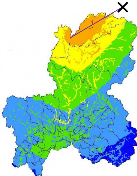
图-9 跡津川断層地震(北東 南)震度階分布
