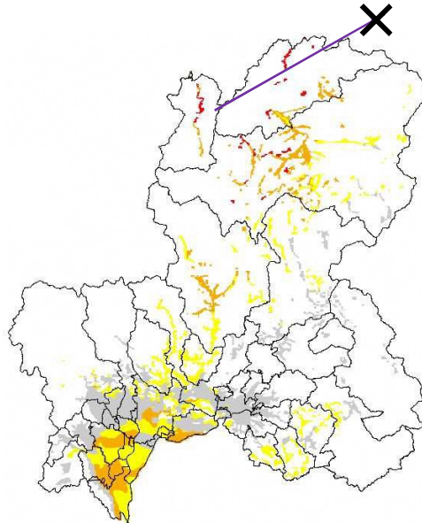
图-20 跡津川断層地震(北東 南)PL 值分布
