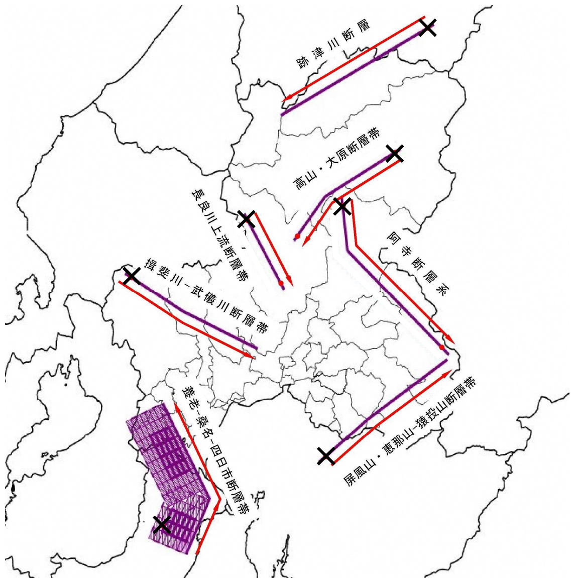
図 1-2 想定震源位置（内陸直下型地震）
