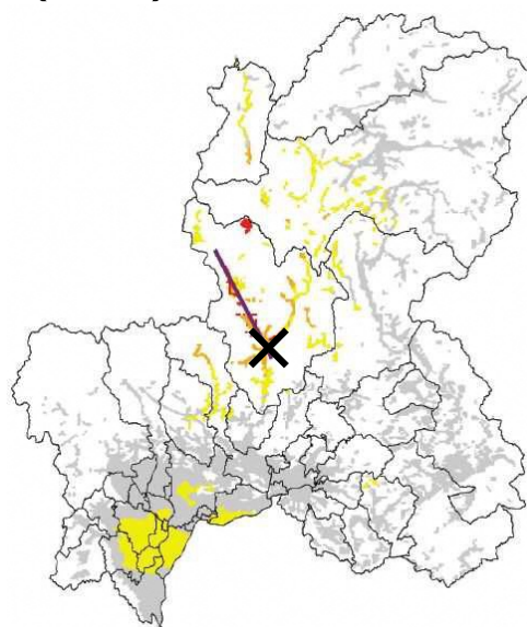
図-16 長良川上流断層帯地震（南 北）PL 値分布
