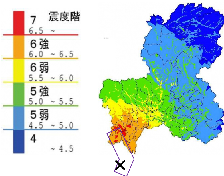
図-3 養老 - 桑名 - 四日市断層帯（南 北）震度階分布
