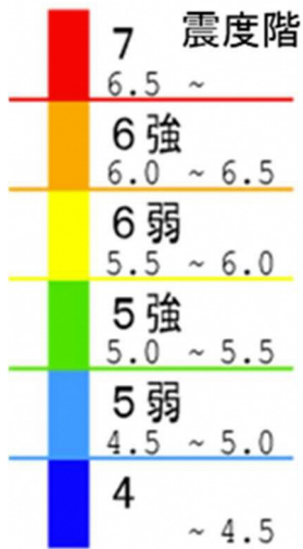
图-7 阿寺断層系地震（北 南東）震度階分布
