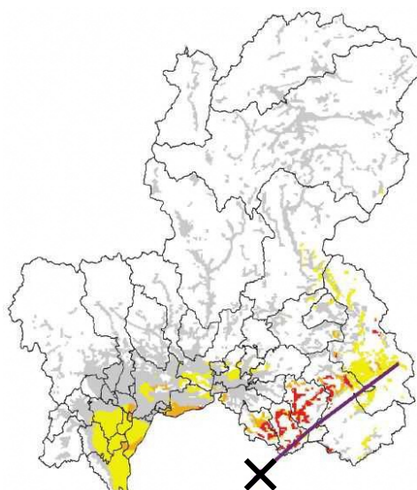
図-17 屏風山・恵那山及び猿投山断層帯地震（南 北東）PL 値分布
