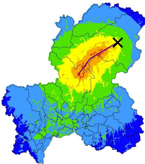
图-10 高山・大原断層帯地震（北東 南）震度階分布
