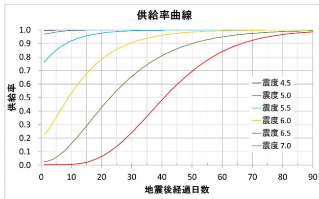
図 2-1 上水道の地震後経過日数と供給率
