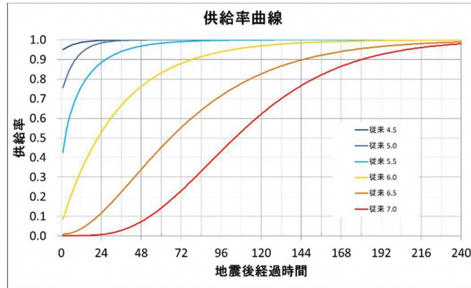
図 2-2 電力の地震後経過日数と供給率
