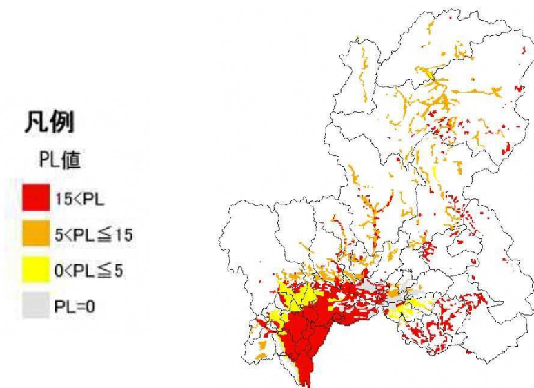
図-12 南海トラフの巨大地震 PL 値分布
