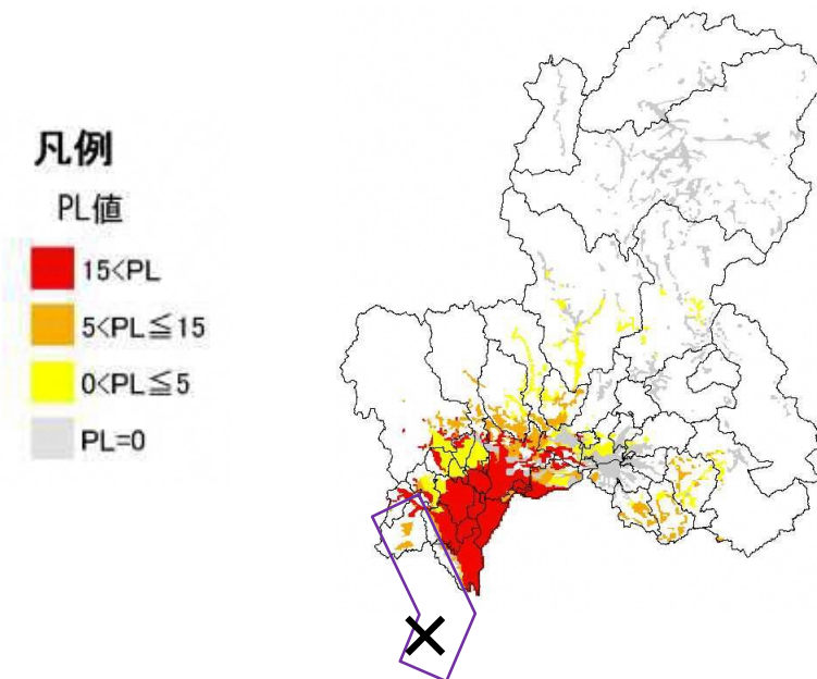
図-14 養老 - 桑名 - 四日市断層帯（南 北）PL 値分布
