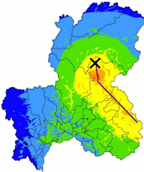
图-7 阿寺断層系地震（北 南東）震度階分布
