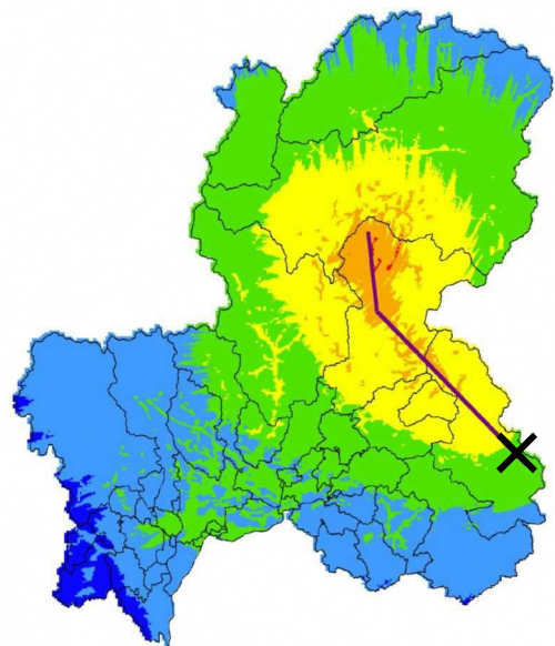
图-8 阿寺断層系地震（南東 北）震度階分布
