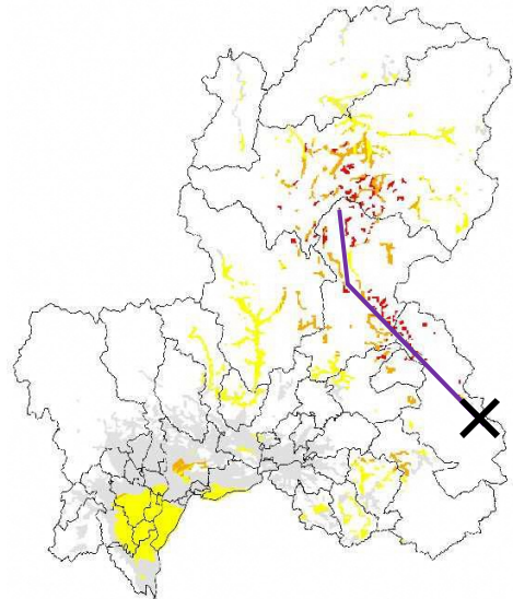
图-19 阿寺断層系地震（南東 北）PL 值分布
