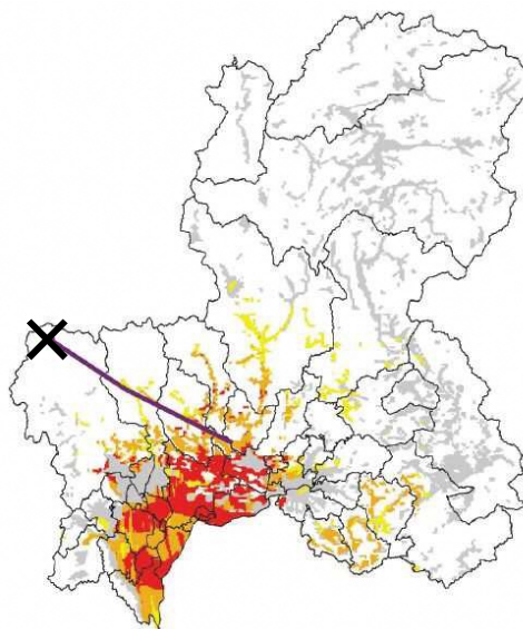
図-13 揖斐川 - 武儀川(濃尾)断層帯地震 (北 南東) PL 値分布
