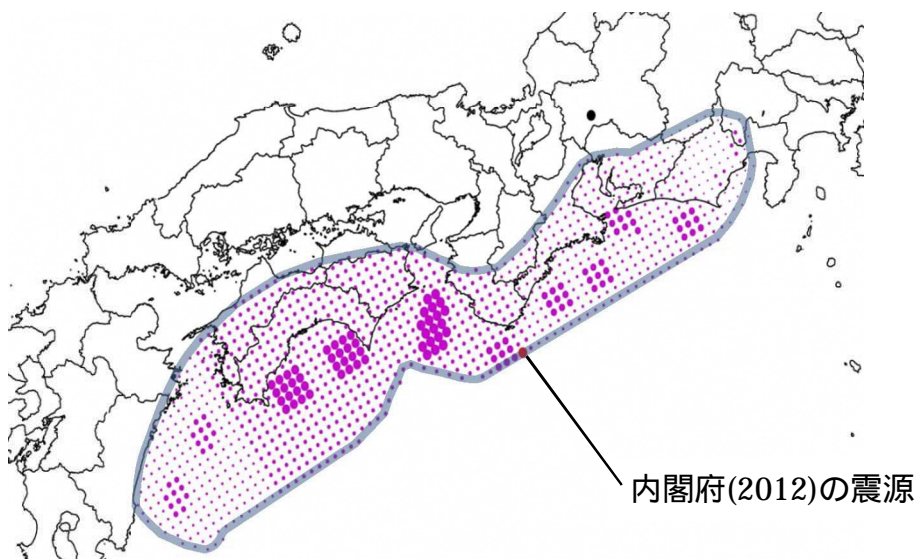
図 1-1 想定震源位置（内閣府（基本ケース））
