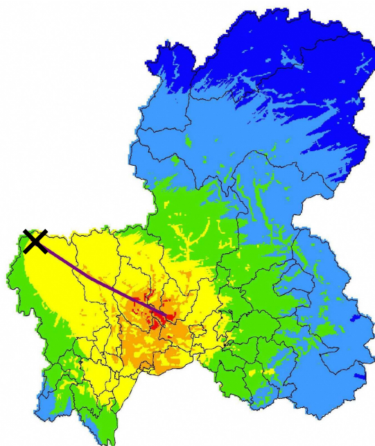
図-2 揖斐川 - 武儀川(濃尾)断層帯地震(北 南東)震度階分布
