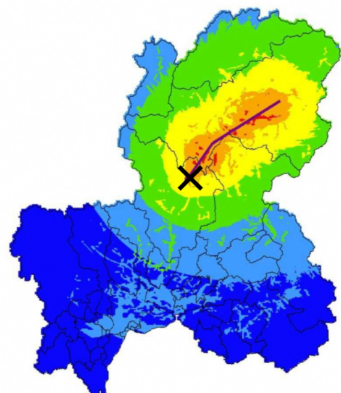
图-11 高山・大原断層帯地震（南 北東）震度階分布
