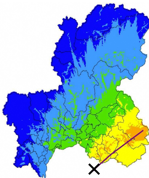
図-6 屏風山・恵那山及び猿投山断層帯地震（南 北東）震度階分布
