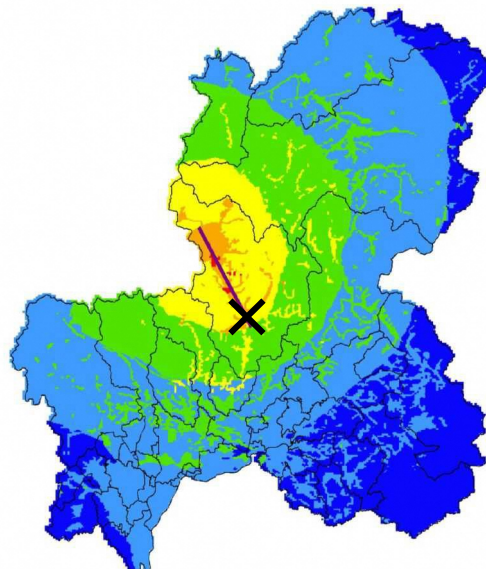
図-5 長良川上流断層帯地震（南 北）震度階分布
