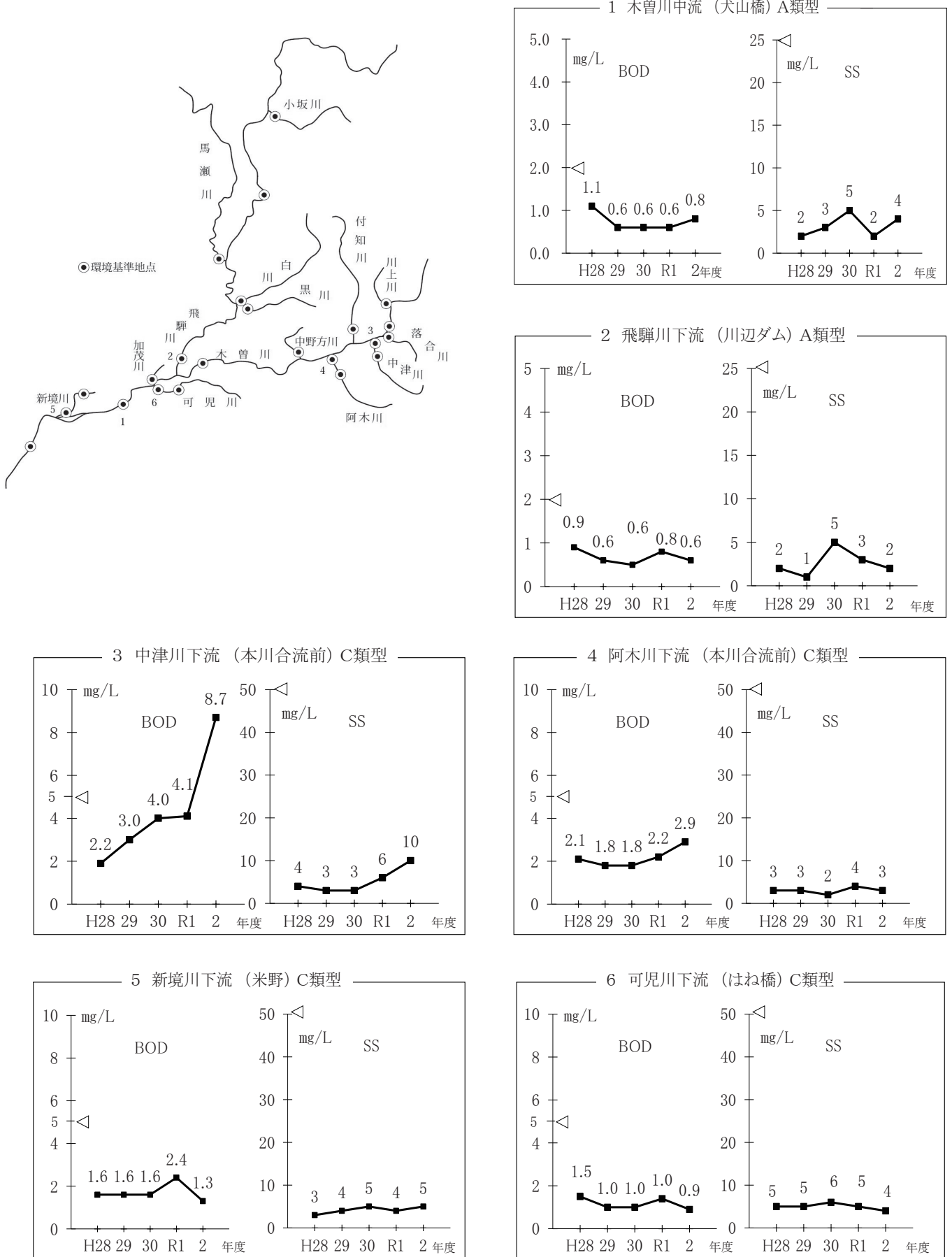
図2-5-2 木曽川水域の主要河川におけるBOD及びSSの経年変化
