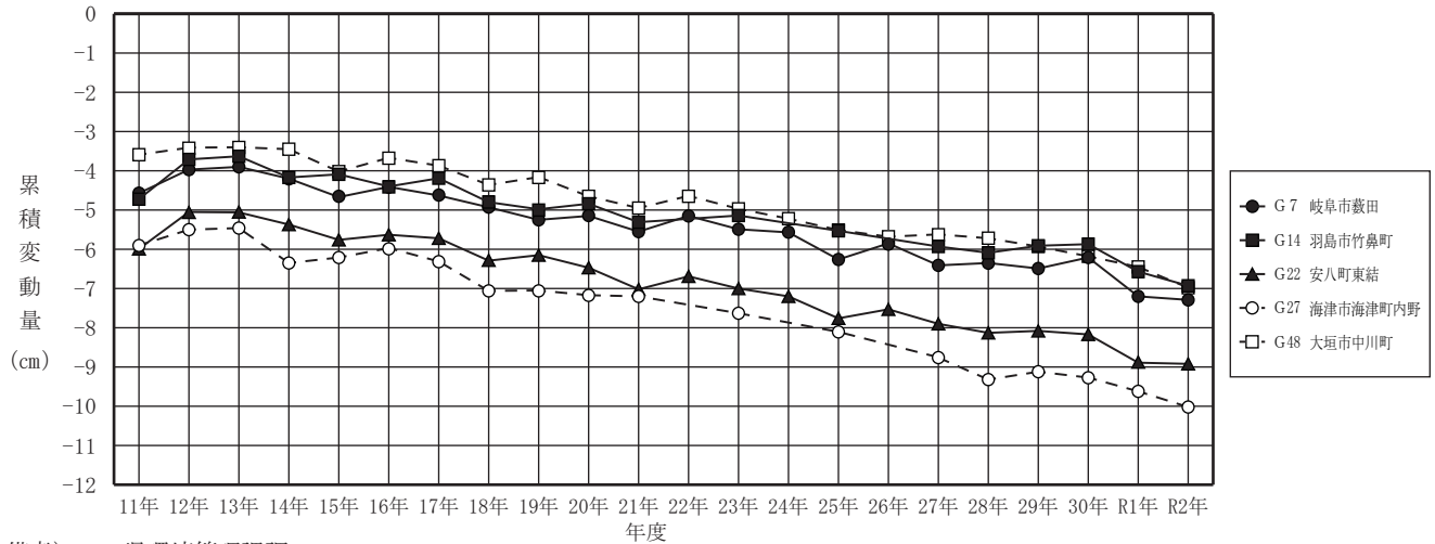
図2-5-22 主要水準点の累積変動量の経年変化
