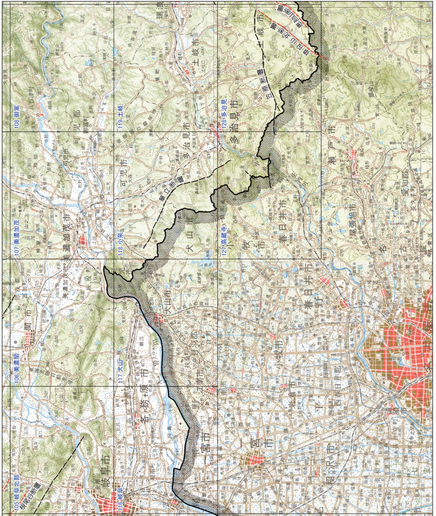
1:25,000 岐阜県活断層図 (縮小版)
