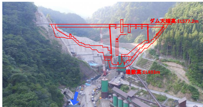
② ダムサイト状況(下流上空より望む)
