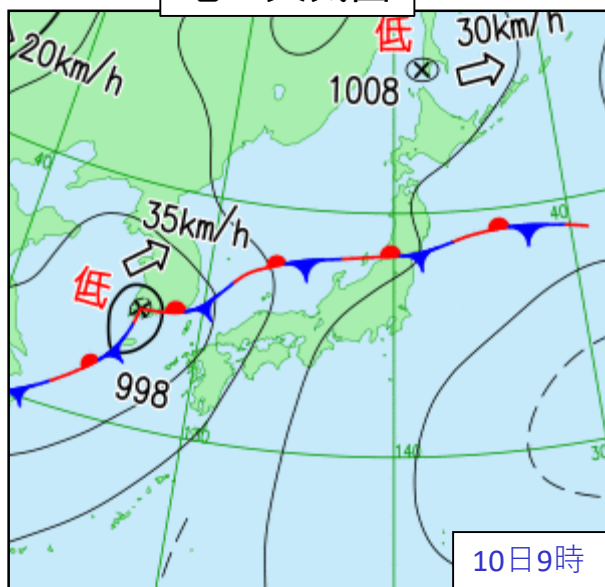
地上天気図
