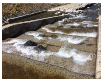
付け石が脱落してしまった魚道 【牛道川(郡上市)】
