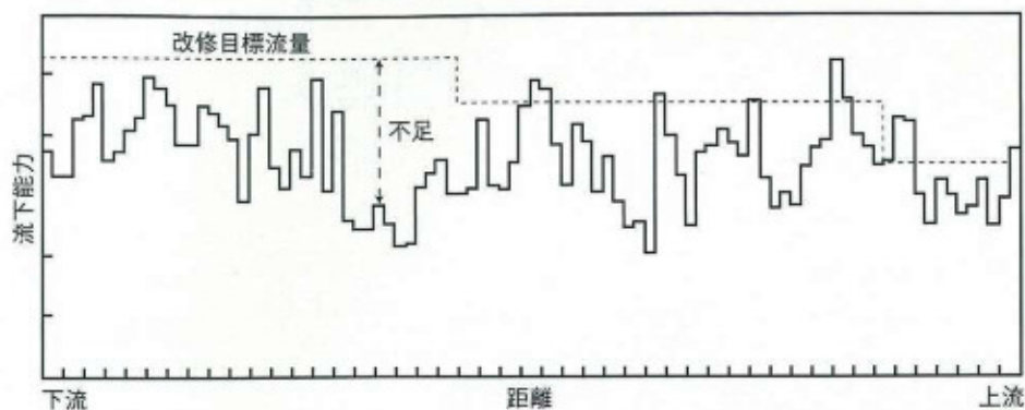
図2-33 流下能力図
