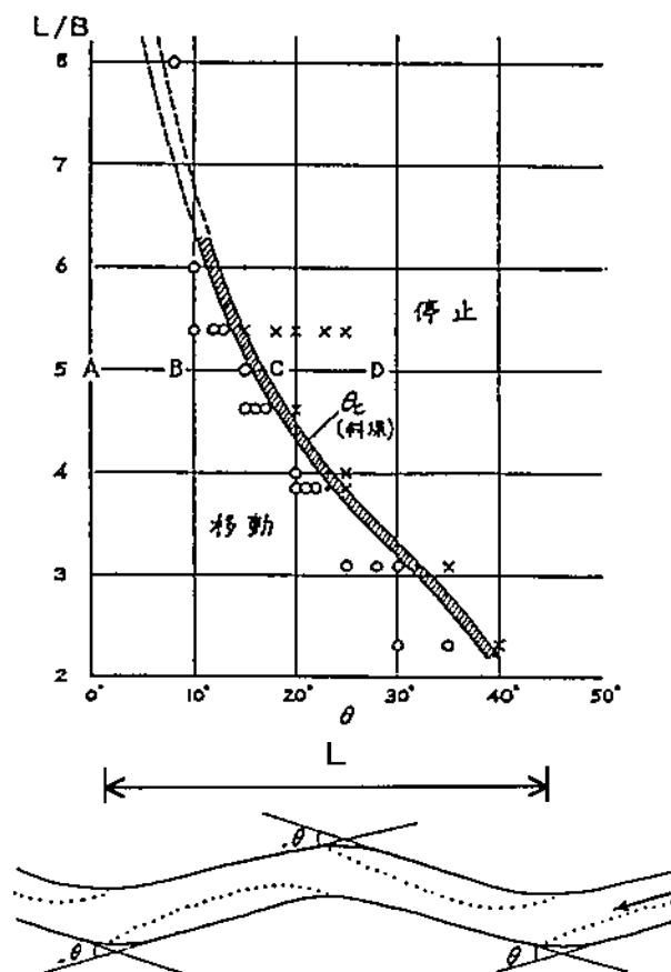
図 砂州の停止限界角度 \theta_c (中小河川における多自然型川づくりより)
