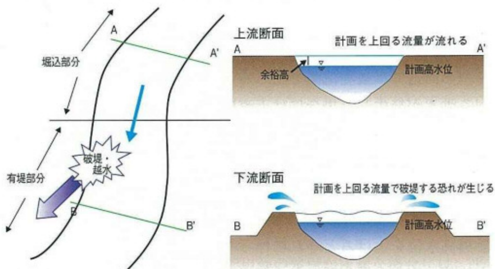
図2-1 堤内地盤高を下回る計画高水位の設定による下流への影響
