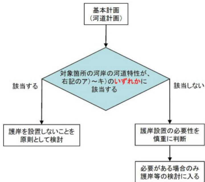
護岸設置の必要性判定フロー
