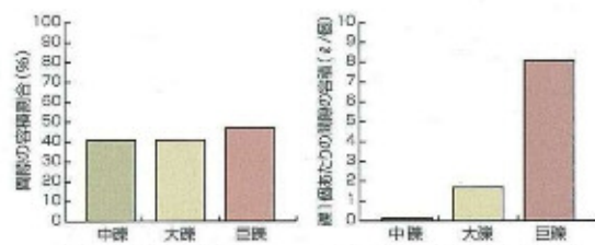
図1 隙間の容積割合
