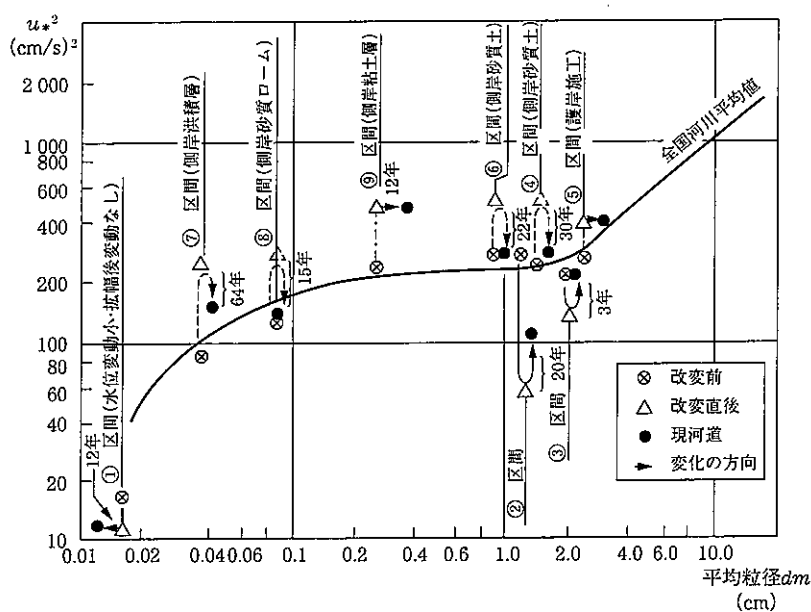
図 7-9 低水路川幅改変に伴う u_*^2 の変化 3)
