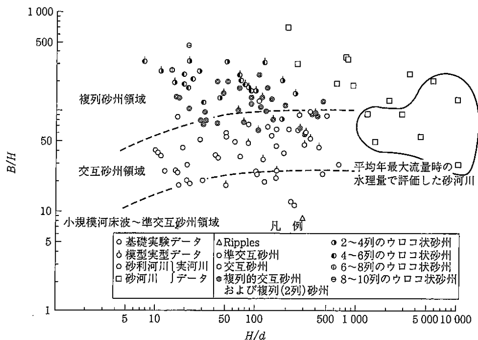
図 7-10 砂州の発生領域区分 3)
