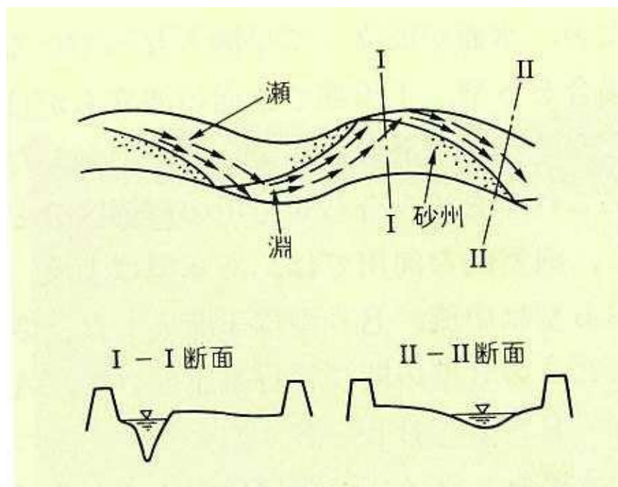
図 砂州と瀬・淵の関係（参考：まちと水辺に豊かな自然をⅡ p18）
