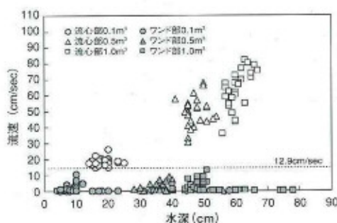
図3 増水に伴う水深および流速の変化
