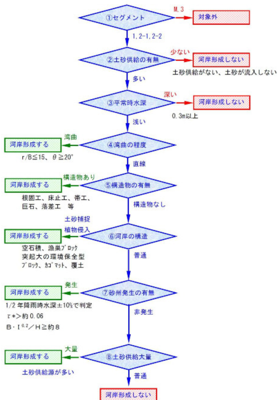
図 3.1.1 対象河川の河岸形成予測フロー
