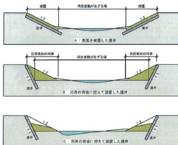
図 4-19 護岸と河岸の区別
