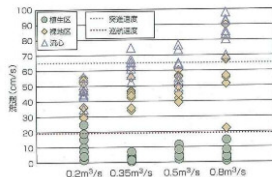
図2 流速推移
