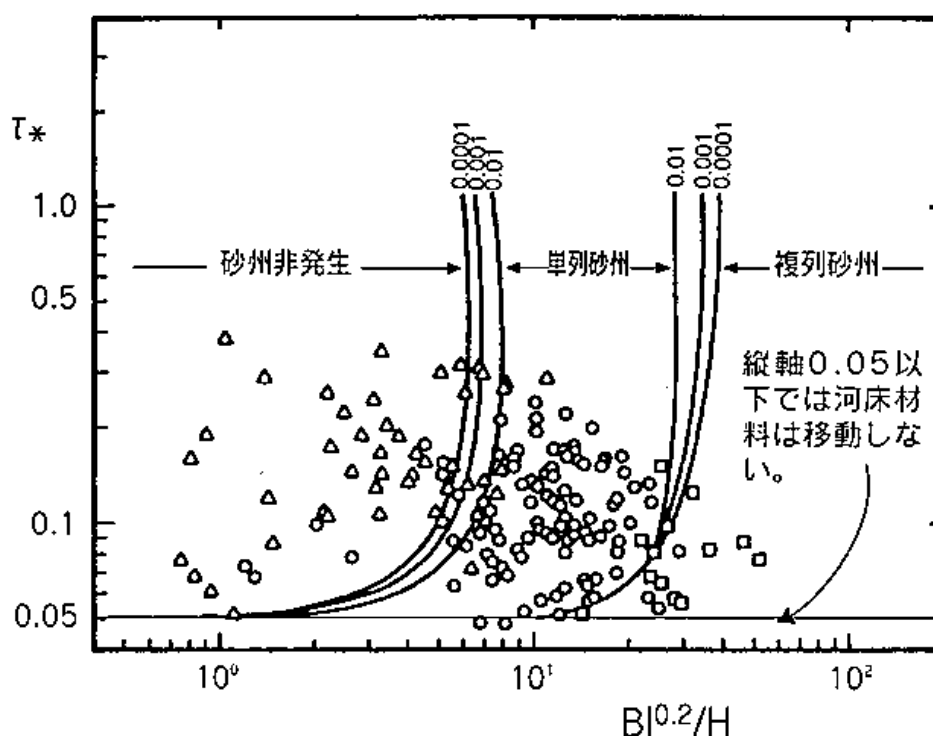
図 水理量の変化と砂州の発生状況(中小河川における多自然型川づくりより)
