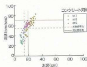
図3 水深・流速分布
