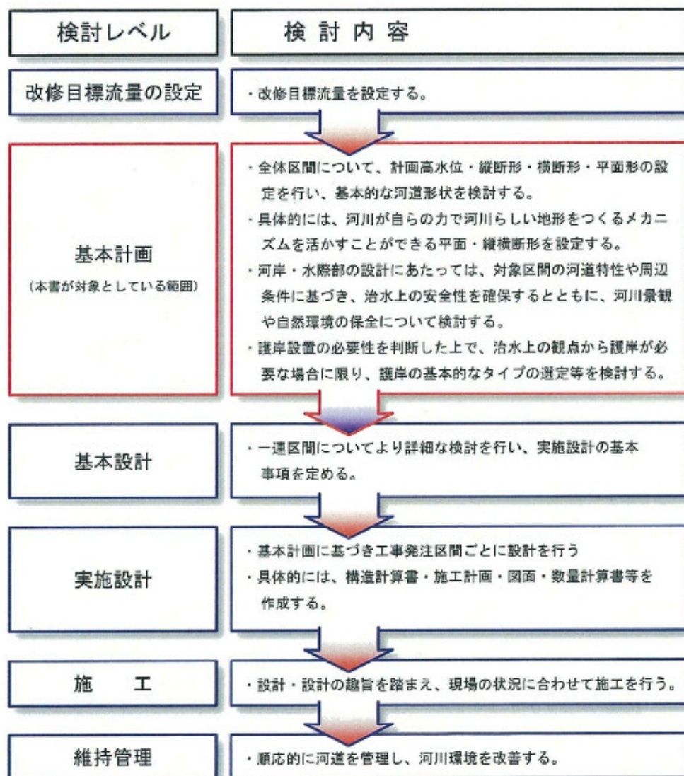
図 1-5 多自然川づくりの流れと本書の対象範囲
