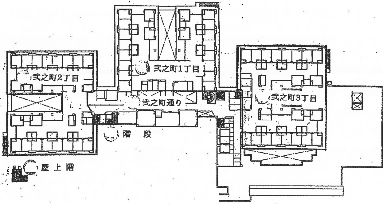
2階平面図
