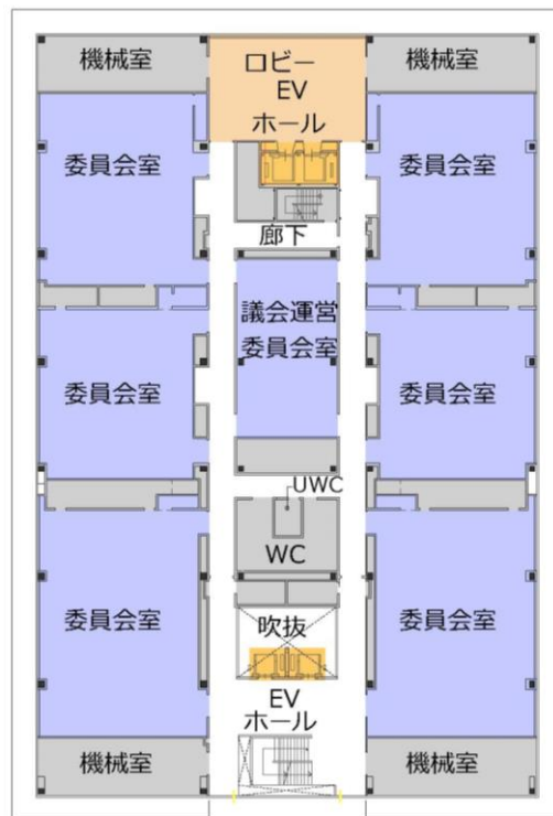
4階平面図
