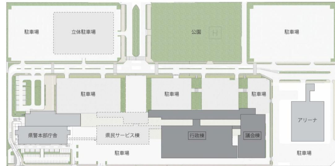
敷地配置図
