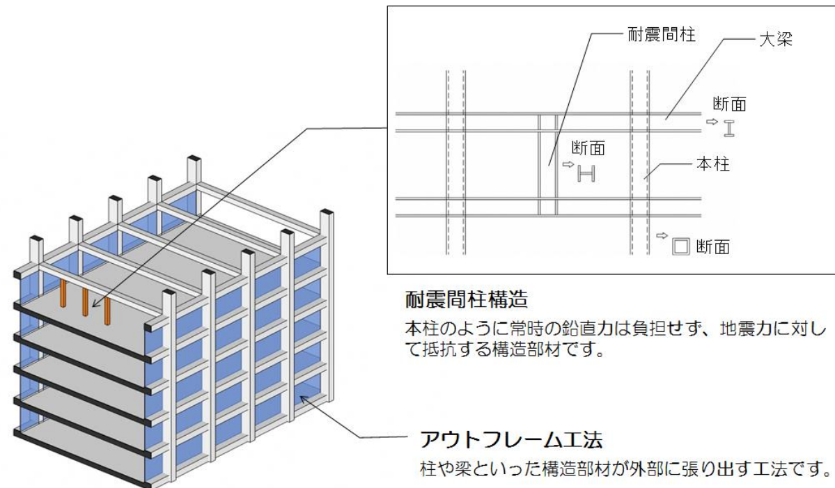
架構計画イメージ図
