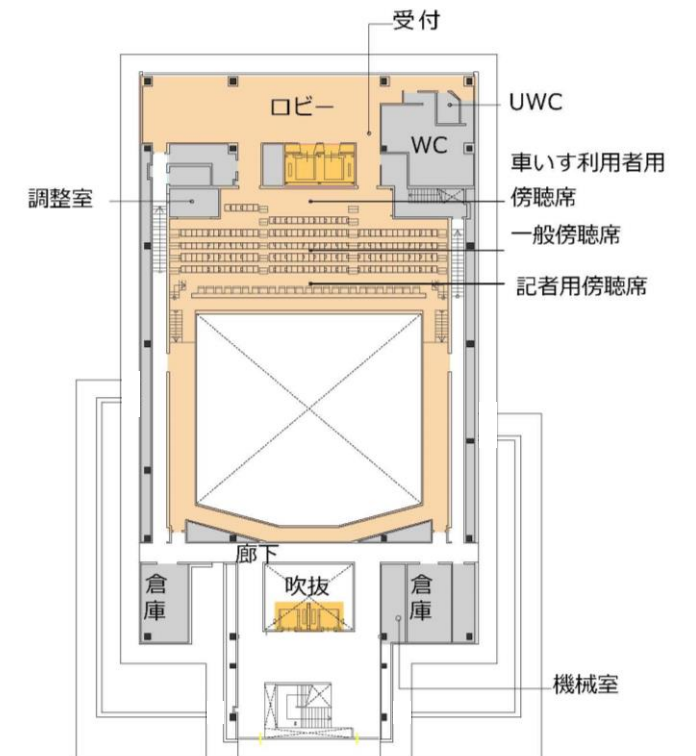
6階平面図
