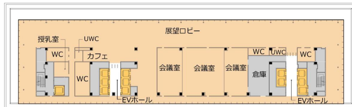
20階平面図
