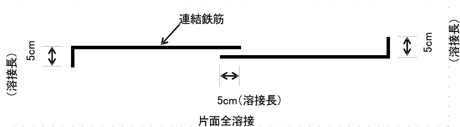
図1-5 コンクリートブロックの鉄筋継手
