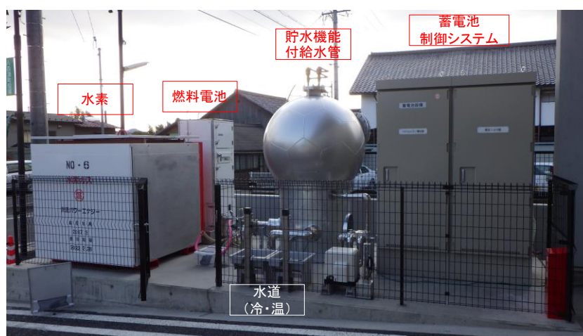
図 資料-17 八百津町の純水素型燃料電池システムの導入状況
