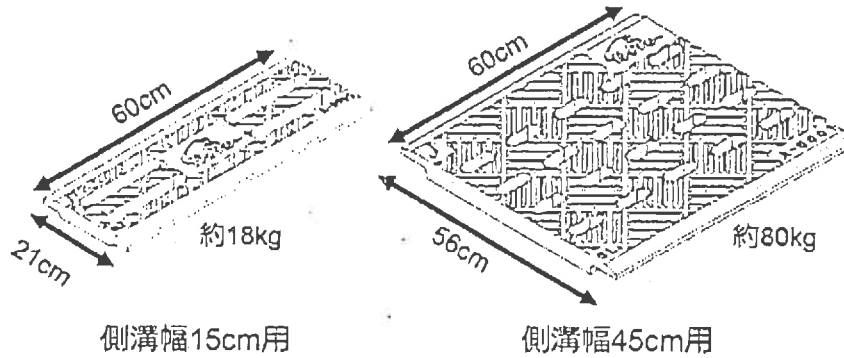
図1 側溝用の蓋(イメージ図)
