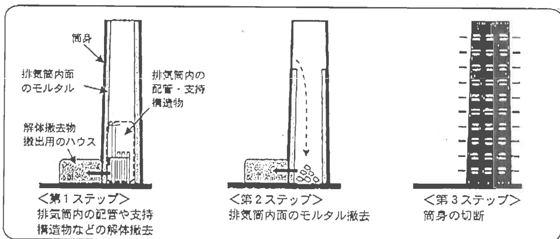
排気筒解体撤去工事の主な工程(イメージ図)
