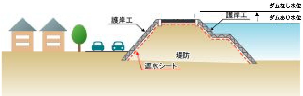
図 3-1 長良川で検討する堤防の形状 (イメージ図)
