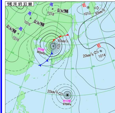
(3日09時) 実況天気図
