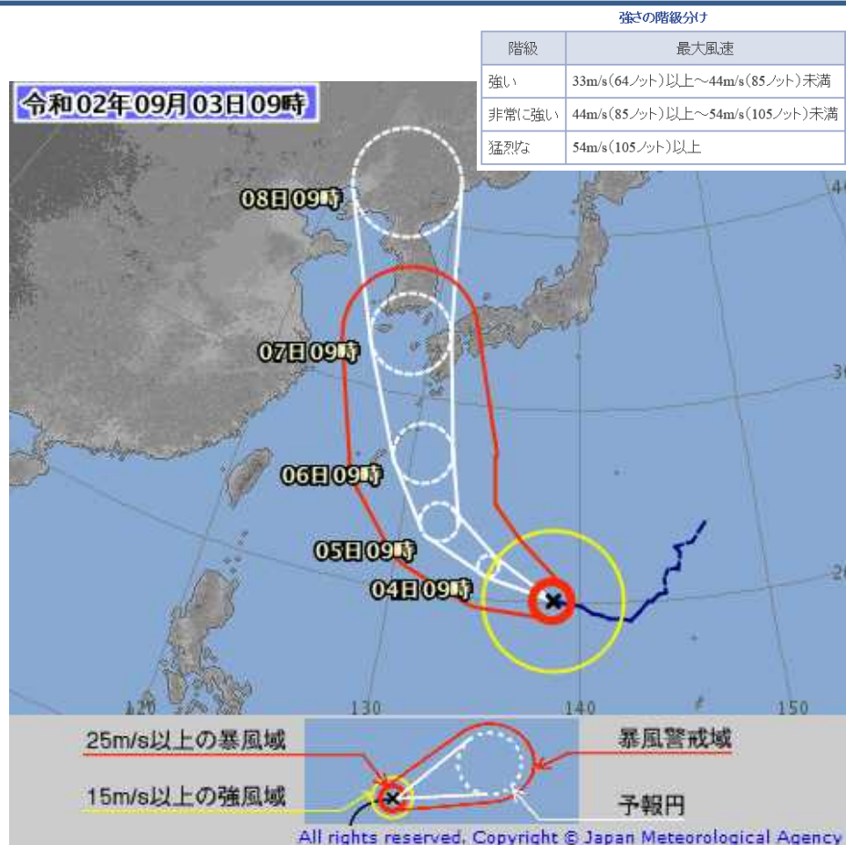
台風進路予想 (9月3日9時現在)
