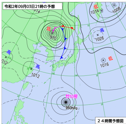
3日21時予想天気図
