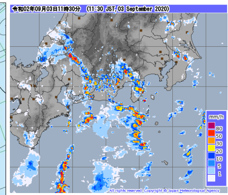
(3日11時30分) 雨雲の様子
