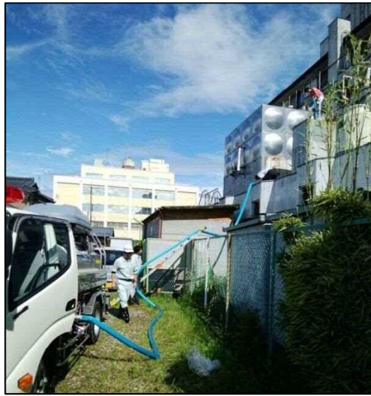
高所受水槽への給水車からの応急給水状況
