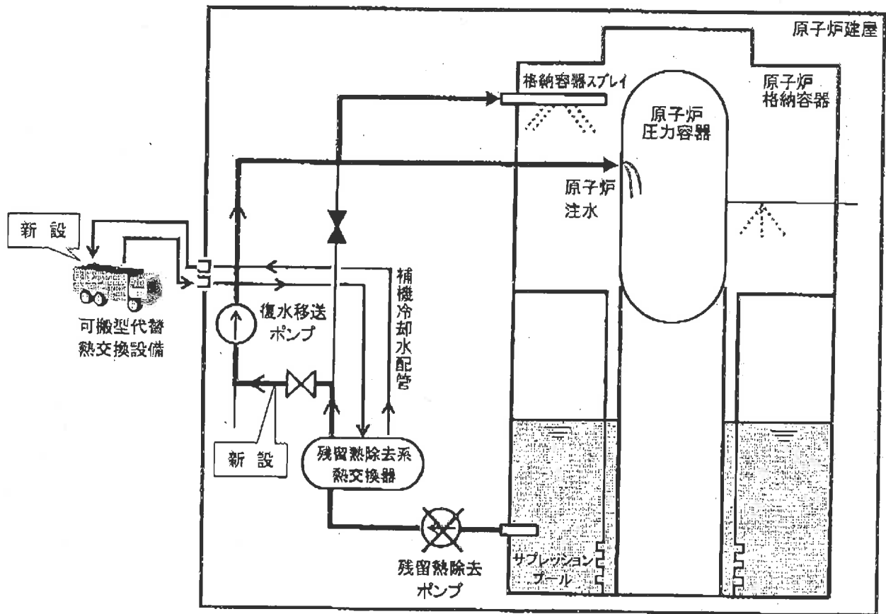
代替残留熱除去設備 系統概略図
