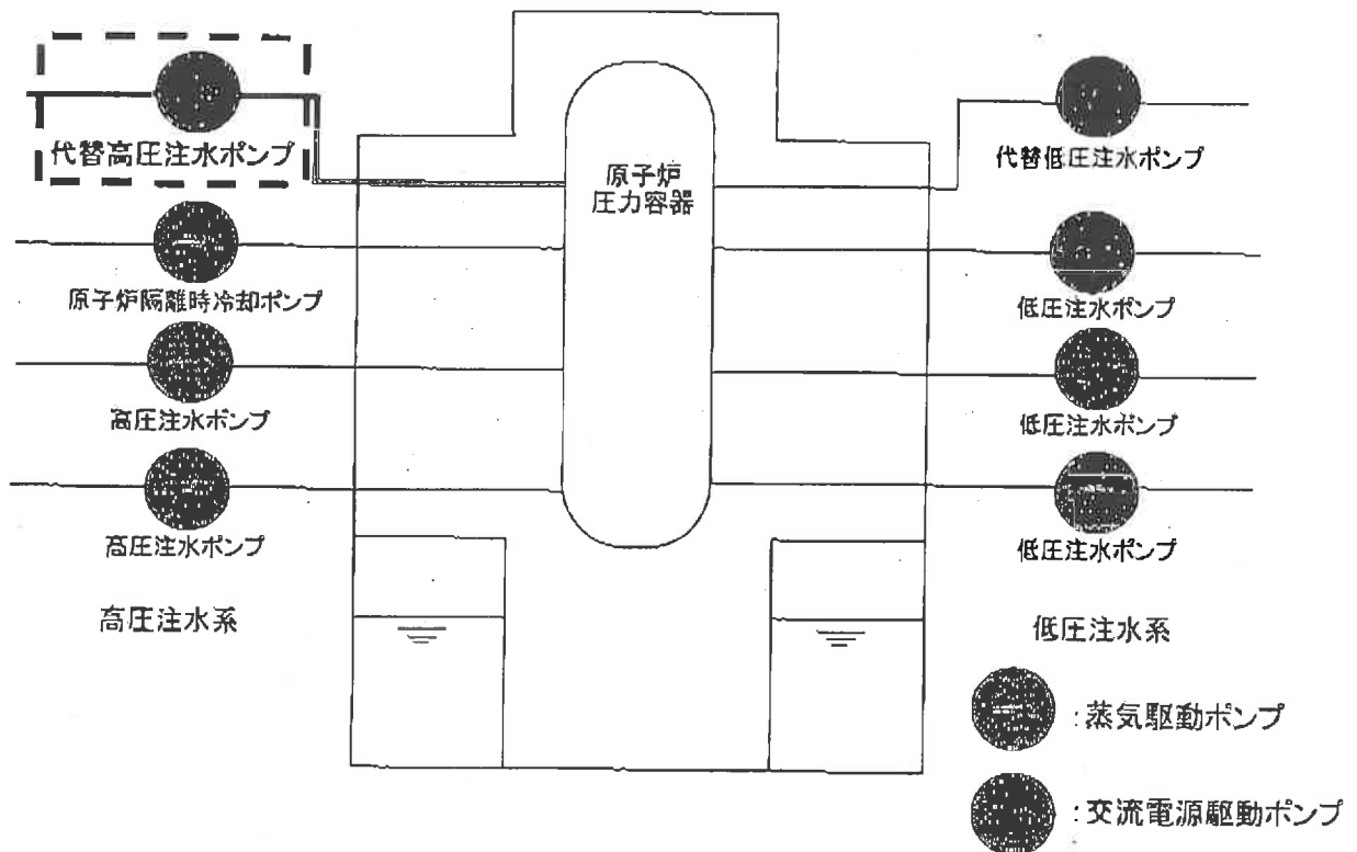
原子炉圧力容器への注水概略図
