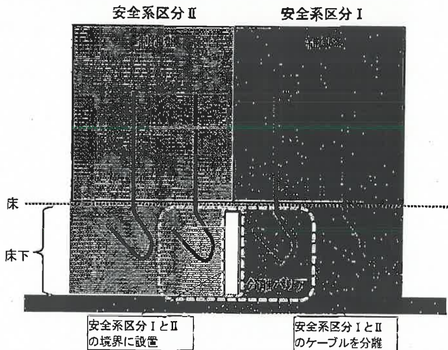
志賀1号機中央制御室ケーブル等敷設状況概要図
